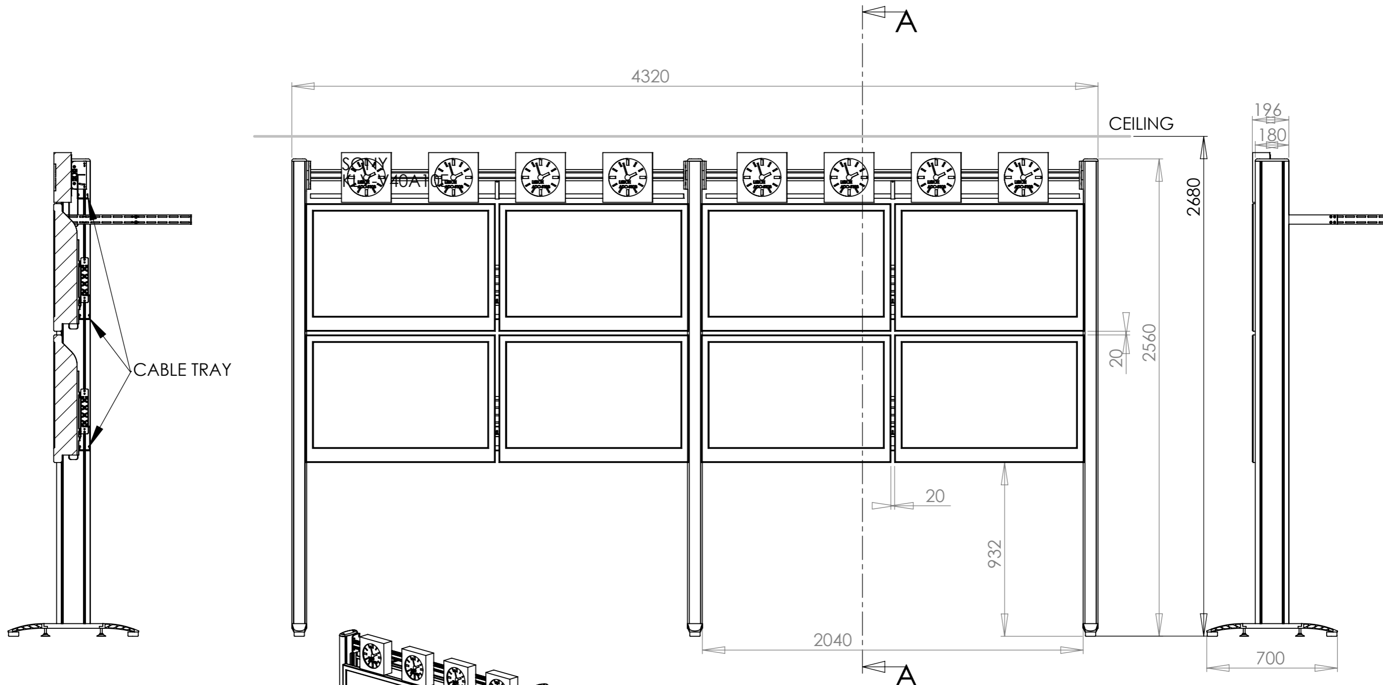
A-A (1 : 20)
